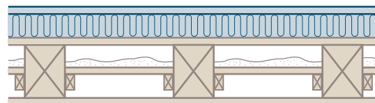
Principskitse - etablering af blændguld: Der udlægges lydæmpende materialer direkte oven på det eksisterende gulv, og herpå udlægges et nyt blændgulv. Kilde: Grundejernes Investeringsfond
