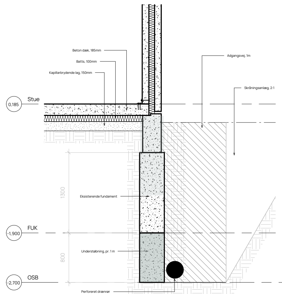
Detaljetejning af understøbning ved eksisterende fundament.
